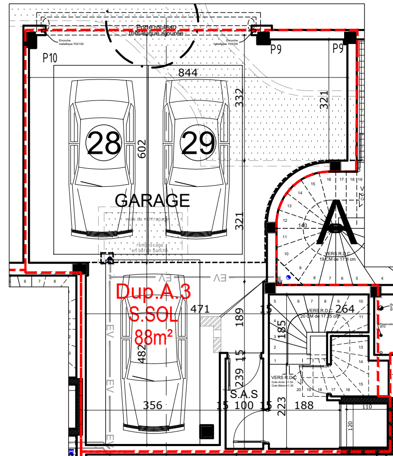
Plan S.SOL
